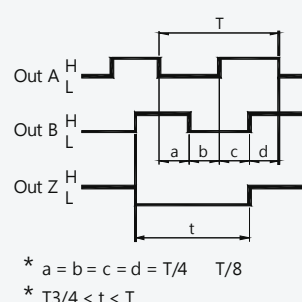
NPN / PNP
